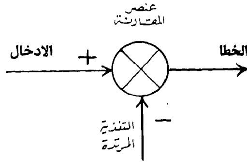
شكل ( ٣ ) عنصر المقارنة في نظام تحكيمي مغلق الحلقة
